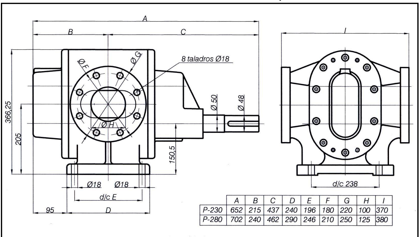
Medidas exteriores de los modelos P-230 y P-280
